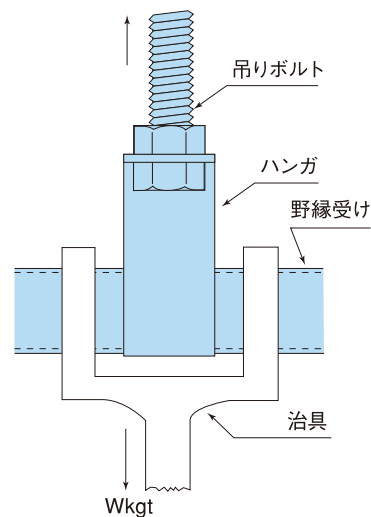
ハンガと野縁受けの組合せ
