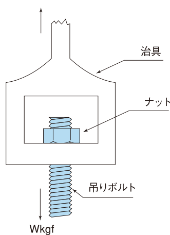
吊りボルトとナットの組合せ
