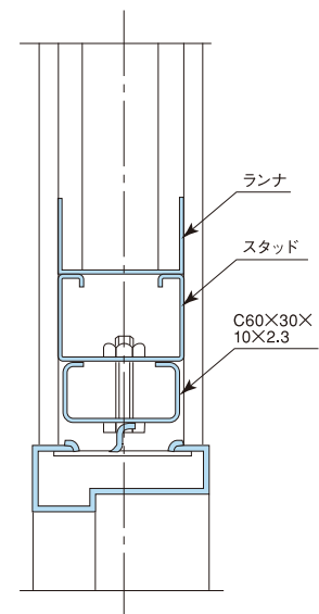
B~B' 断面図
