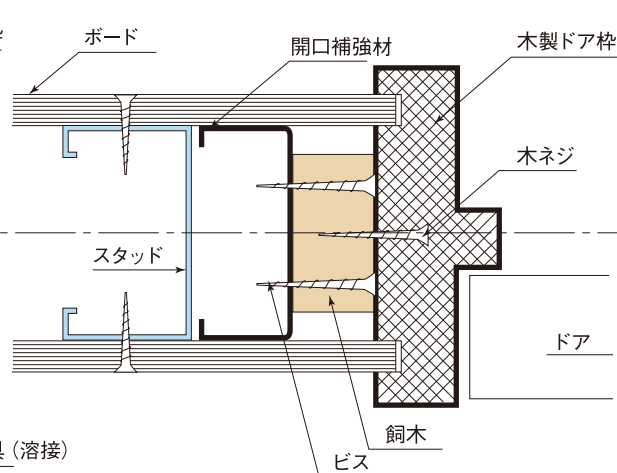
●木製ドア枠取付け
