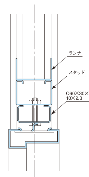
B~B' 断面図
